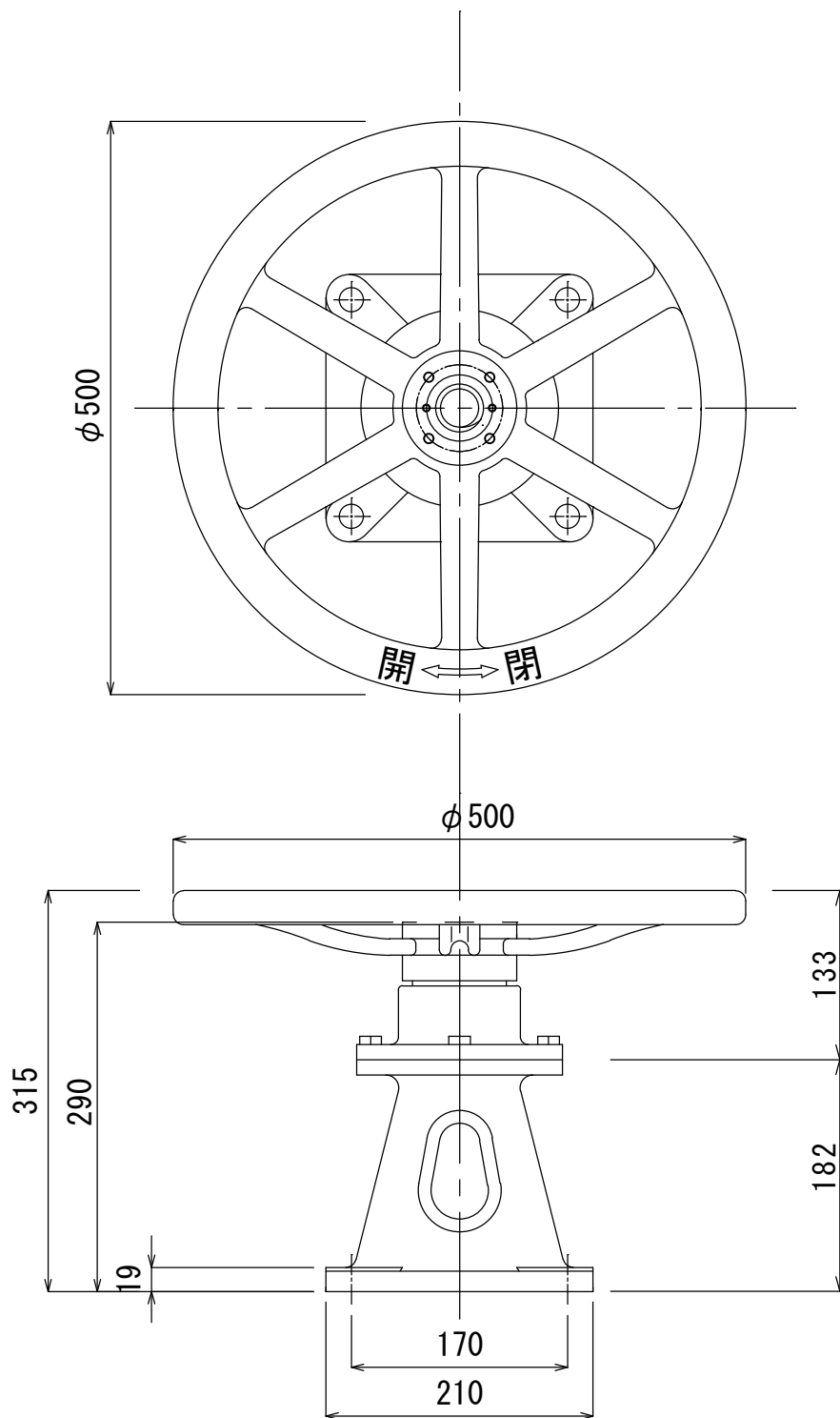
\phi 45 平卷式卷上機 スタンション182mm
