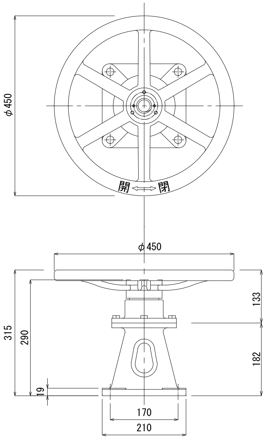
\phi 38 平卷式卷上機 スタンション182mm
